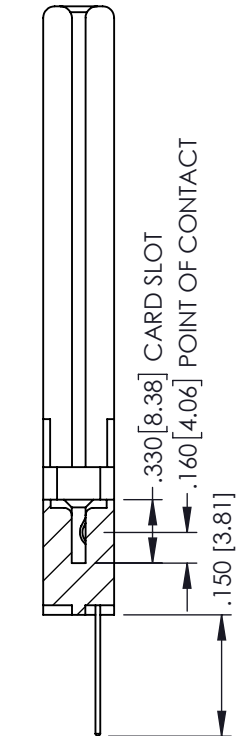
SECTION A-A
