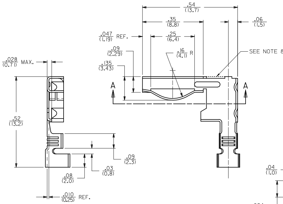
CARRIER STRIP DETAIL ACTUAL SIZE
