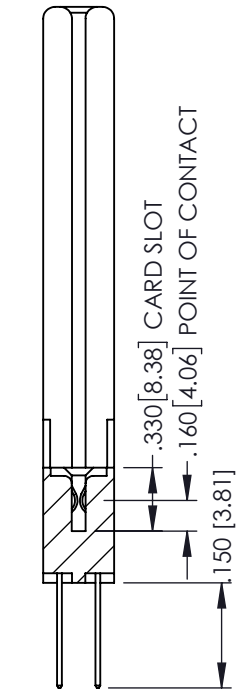
SECTION A-A
