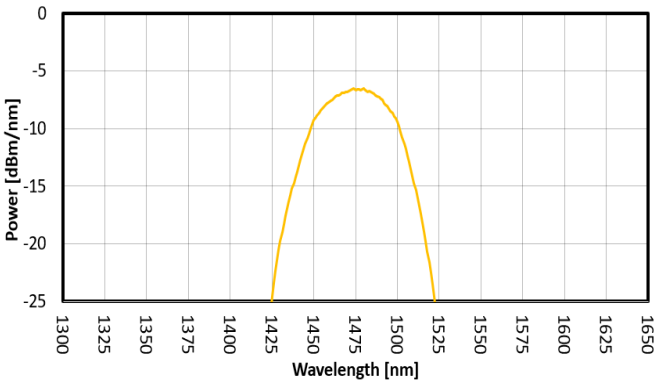
FIG. 3: SLED 2 SPECTRUM
